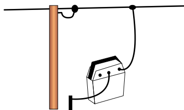
Připojení zdroje impulsů na elektrický ohradník a uzemnění.
